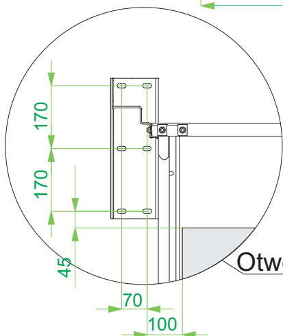
szczegół A widok bez elementów napędu
