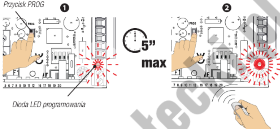
Przycisk PROG
